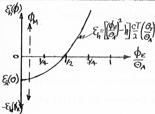
e. - ALTITUDE ERROR VS ATTITUDE
