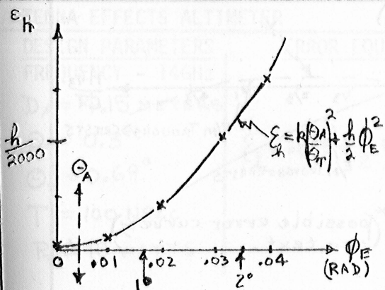
e. - ALTITUDE ERROR VS ATTITUDE
