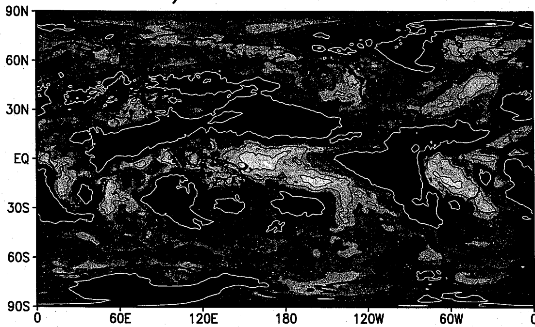
b) Nature run HCC
