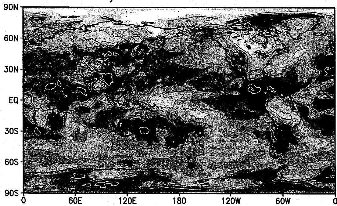
a) Nature run TCC
