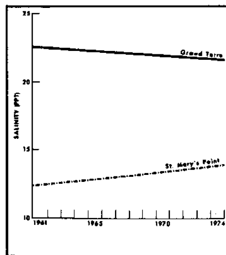
Fig. 6 Linear salinity trends 1961-1974.
