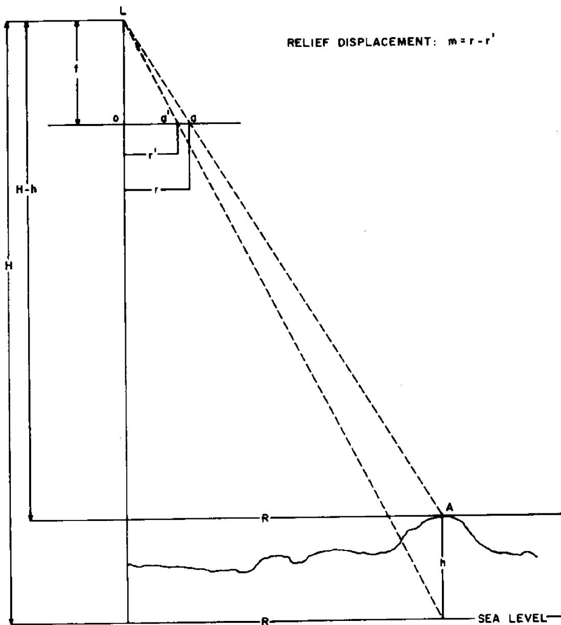
FIG. 4 Relief displacement, (Moffitt, 1967).
