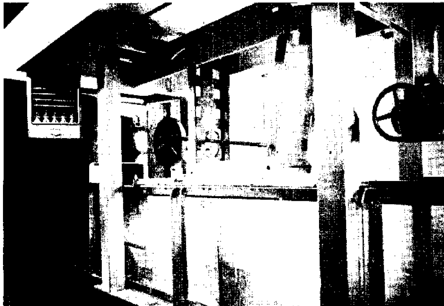
FIG. 4.-WAVE GENERATOR
