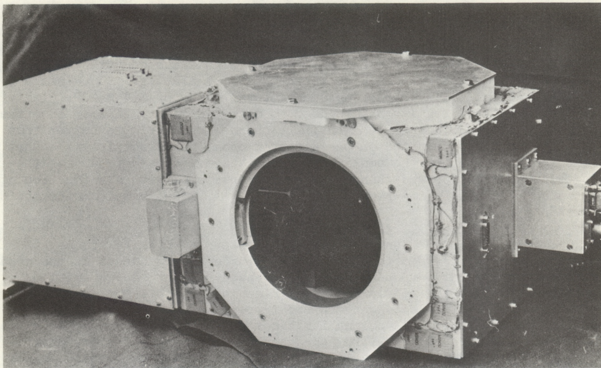
Figure II-4.--ITPR optics unit.
