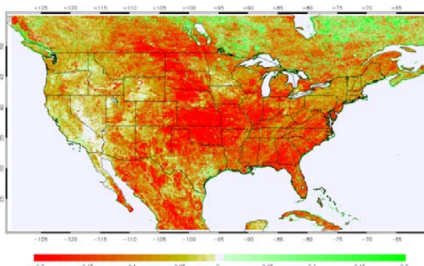
VIIRS GVF anomaly (15 August 2012)
