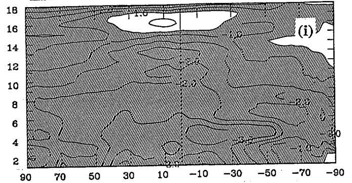
LHW FT=24 JJA 1990
