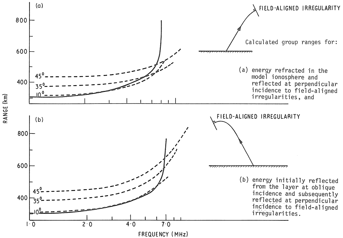
Fig. 2.17
