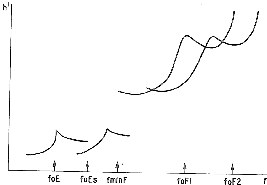
Fig. 3.6 Lacuna Case
