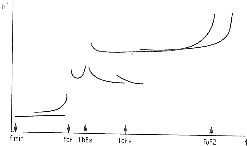
Fig. 4.20 Non-blanketing Es.
