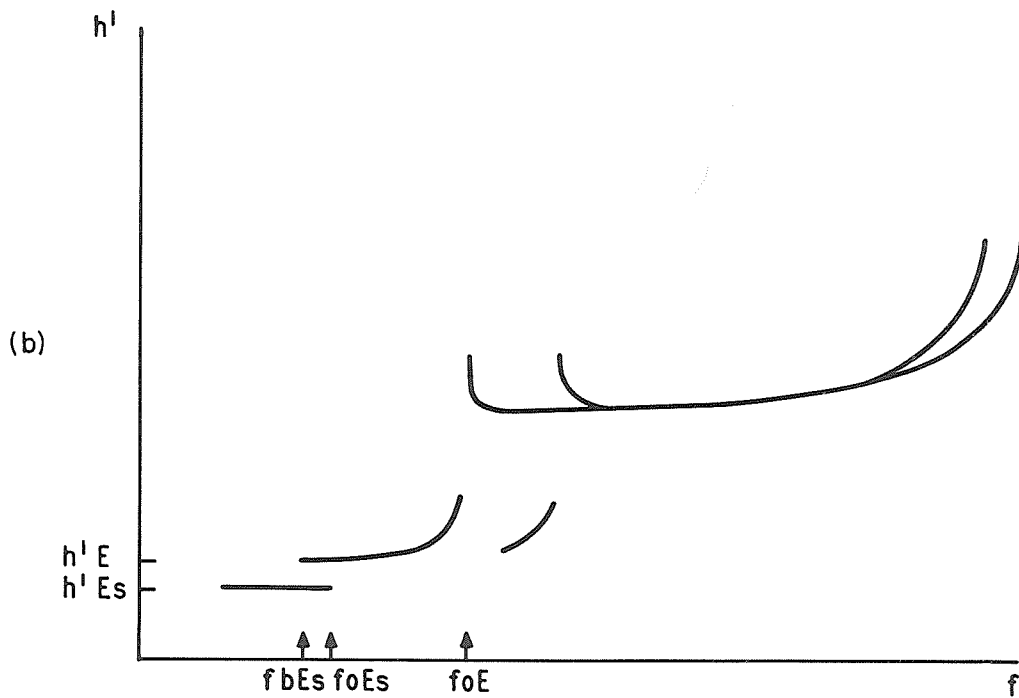
Fig. 4.24 (a)(b) Es type l , low
